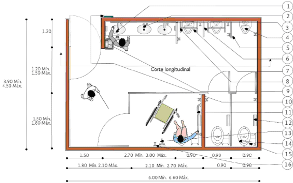
Planta: Sanitarios para hombres.
