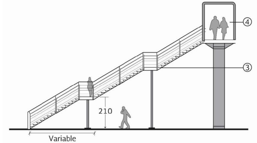
39 ALZADO DE PUENTE PEATONAL
