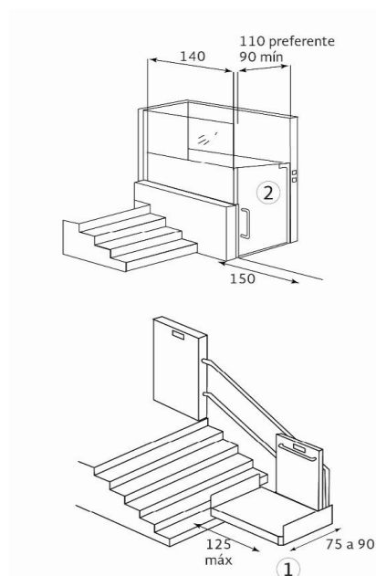
61 ISOMÉTRICO DE PLATAFORMAS/SALVAESCALERAS
